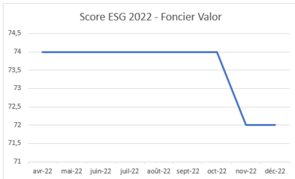
Figure 1 : Évolution de la note ESG du fonds au cours de la période de référence
